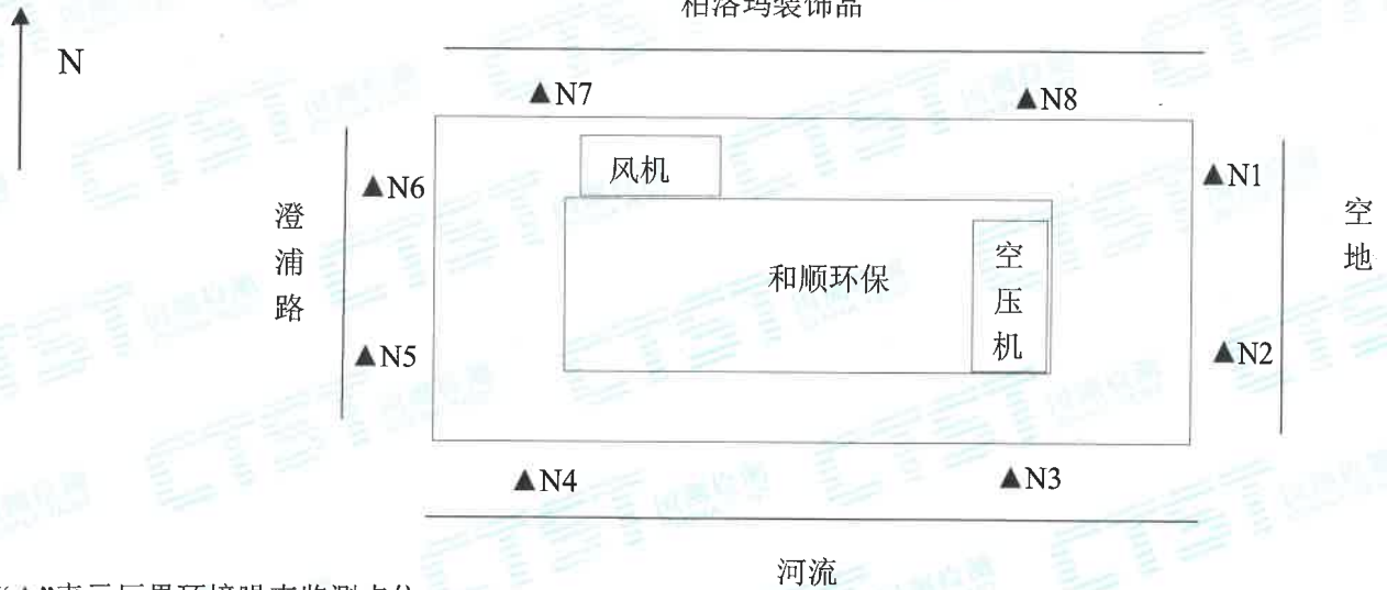
测点示意图:
