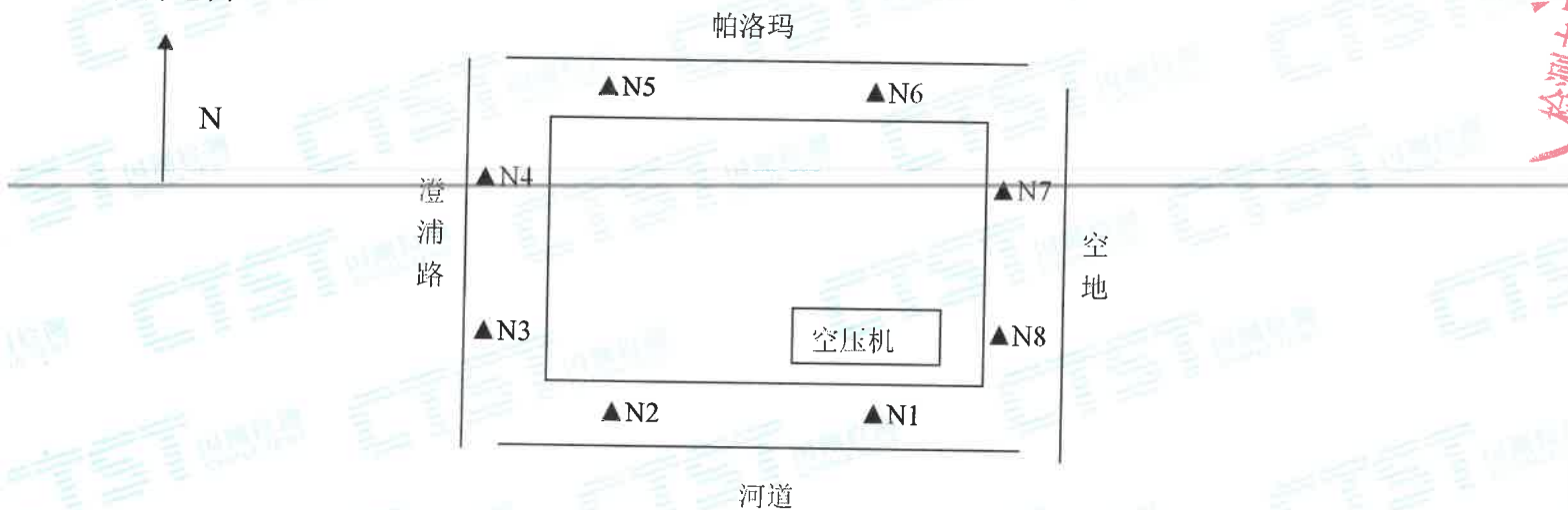
测点示意图:
